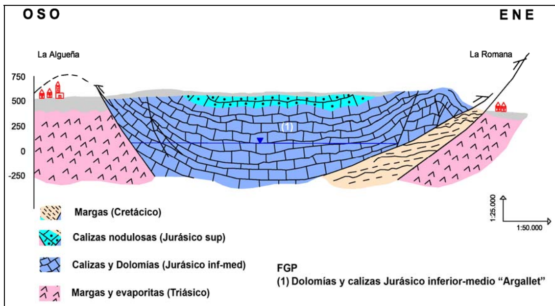
Figura 2. Corte esquemático I-I' del acuífero de la Sierra de Argallet.
