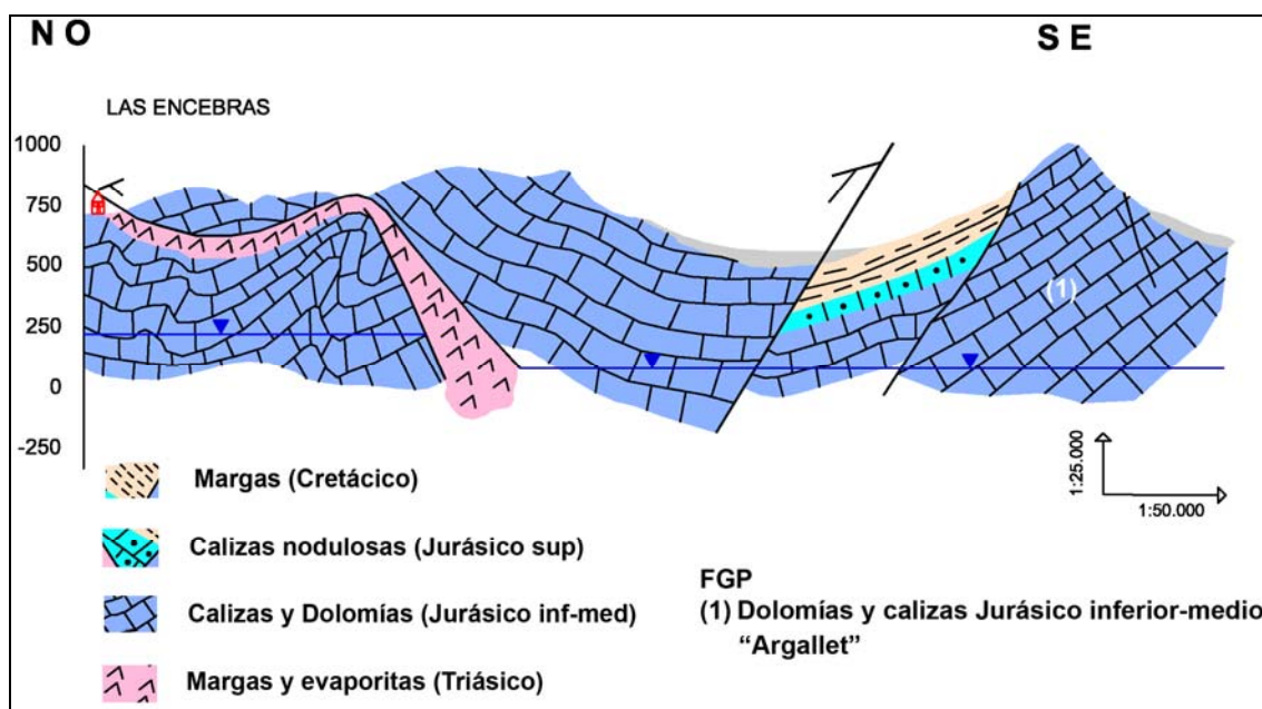
Figura 3. Corte esquemático II-II' del acuífero de la Sierra de Argallet.
