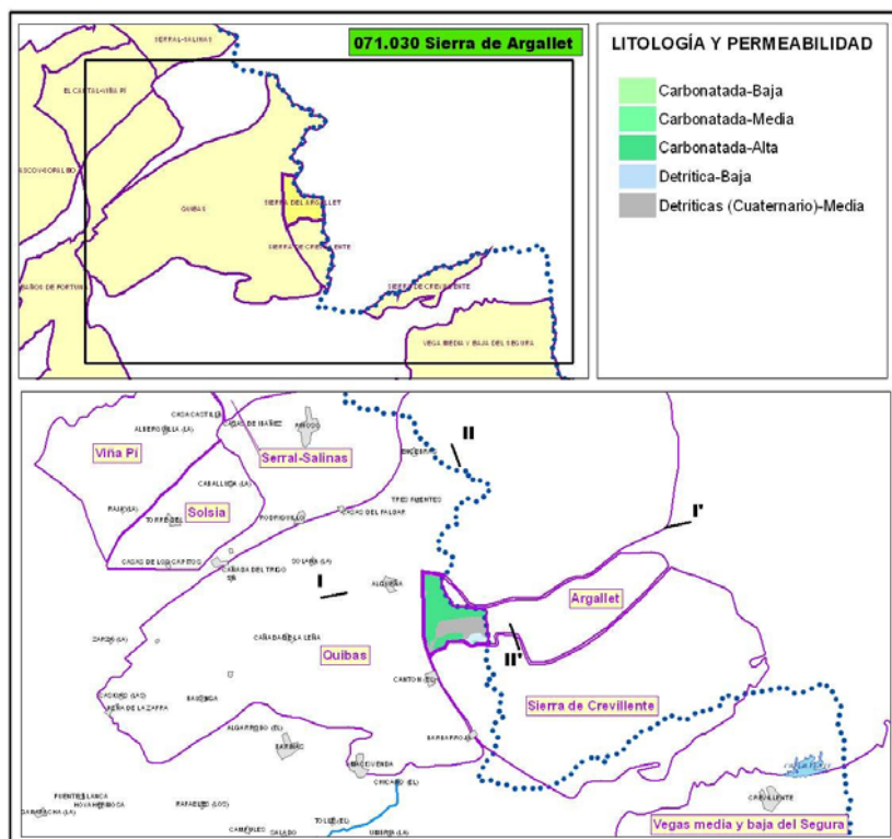
Figura 1. Mapa de situación de cortes del acuífero de la Sierra de Argallet.
